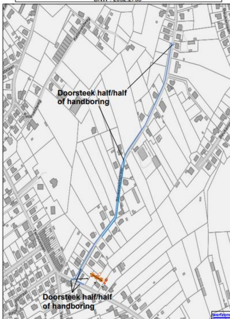
Signalisatieplan: Hoeilaart – Sloesveldstraat DNW : 2032.2733
